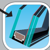
Vidrio laminado y anti intrusión clase P2 – composición de vidrio: vidrio exterior templado y capa de fácil limpieza y el vidrio interior laminado. El interior relleno con gas noble. Marco aislante TGI.
